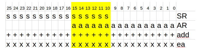
Abbildung 1: Überlappung der Register
