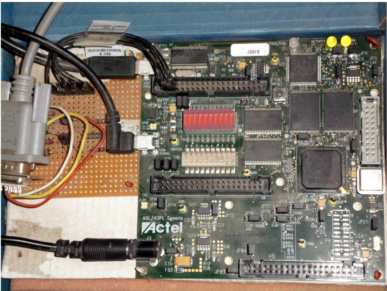
Abbildung 2: Der STRIP-Prozessor im Evaluation-Board; links oben die RS232-Schnittstelle.
